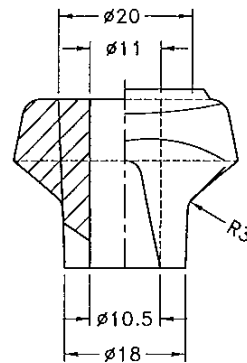
Section : C-E
